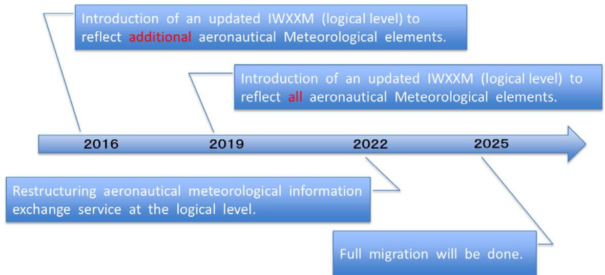
圖 7、IWXXM 計畫圖
