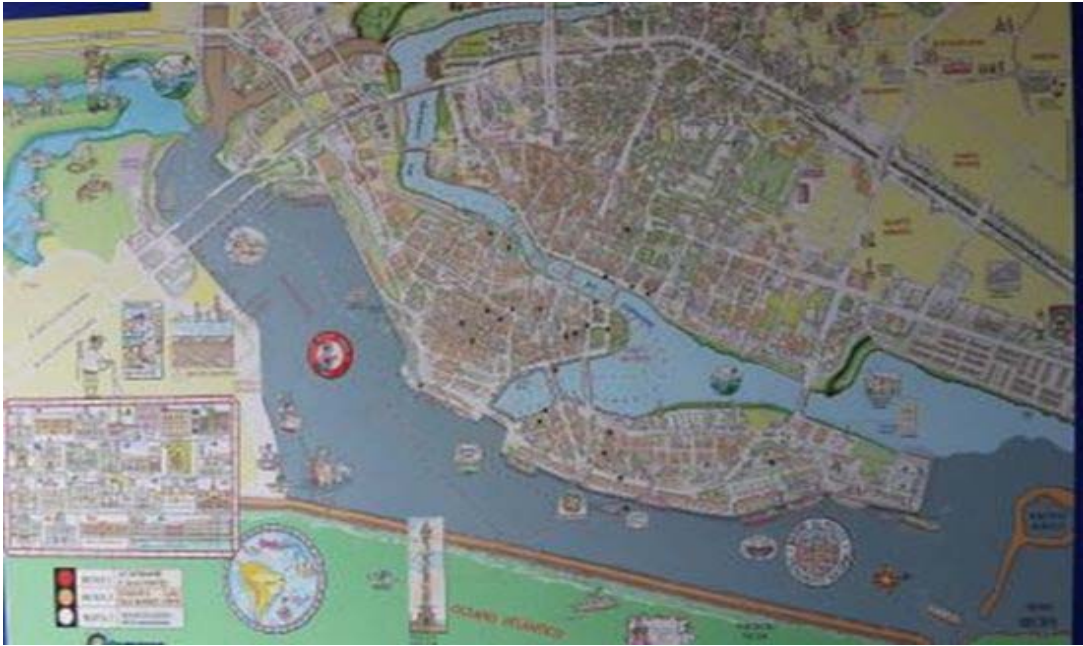
IOJT第七屆年會舉辦地瑞西費市地圖
