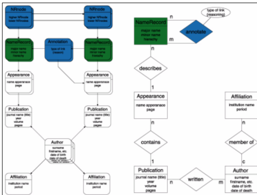
圖七 Nomencurator Data Model
